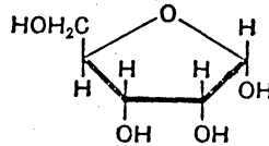
\alpha -D-Ribofuranose
