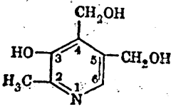
Pyridoxine
