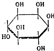
meso-Inositol
